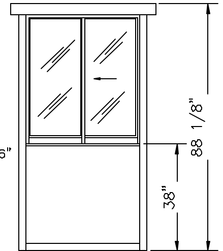
ELEVATION B
