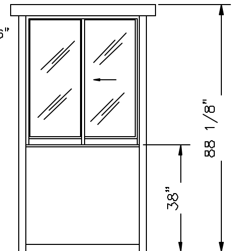
ELEVATION B
