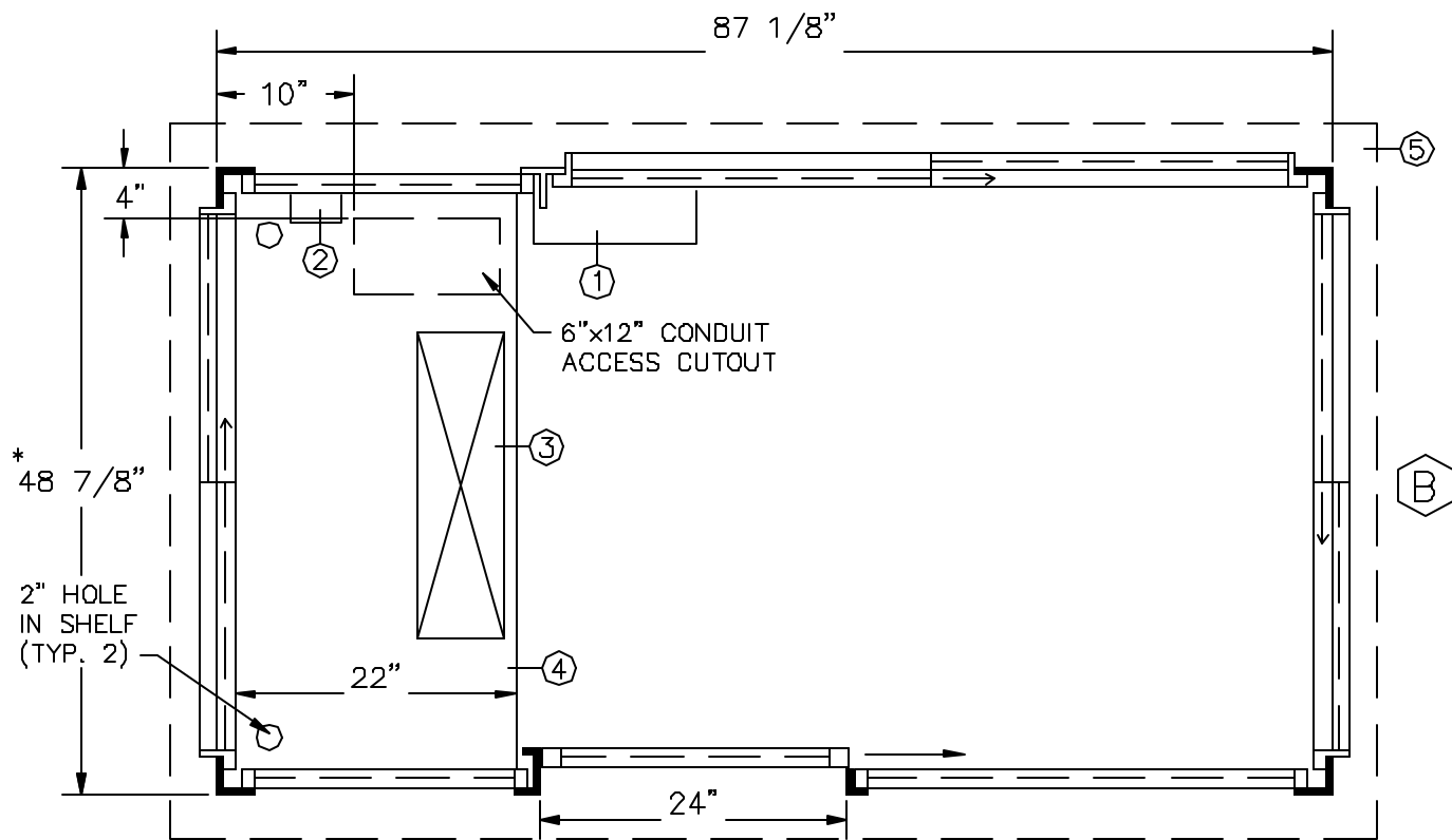
A PLAN VIEW (N.T.S.)
