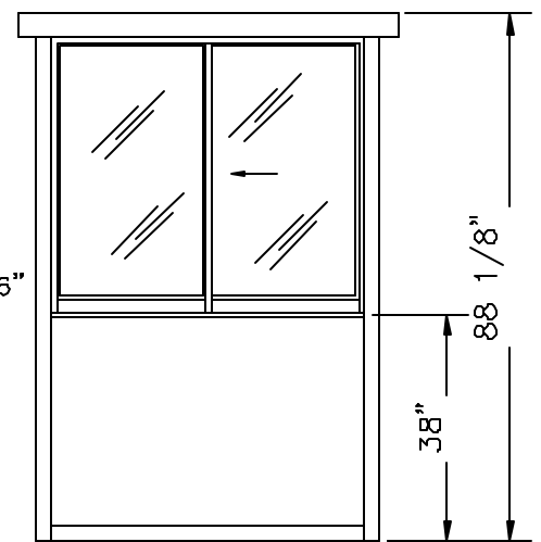
ELEVATION B
